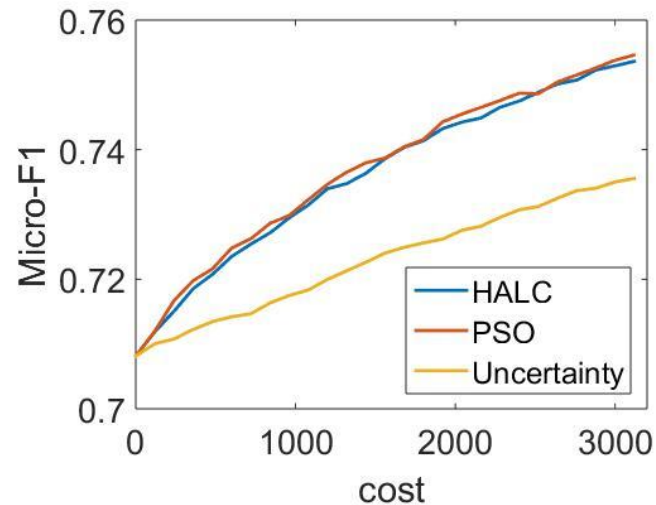
ImageCLEF07A
