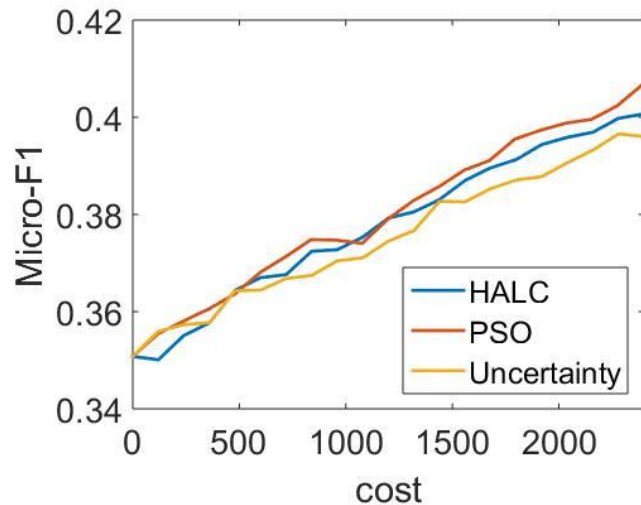
ImageCLEF07D
