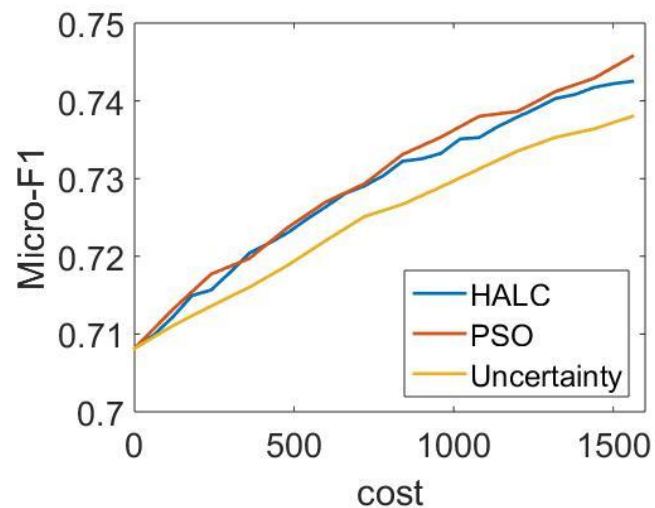
ImageCLEF07A
