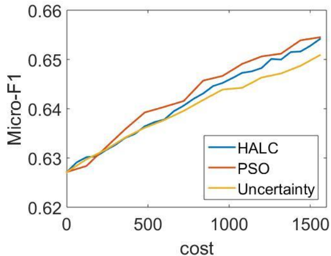
ImageCLEF07D
